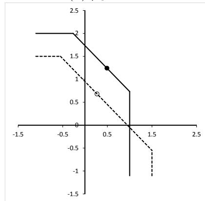
(d) \rho_F = -0.5, \rho_G = -0.8
